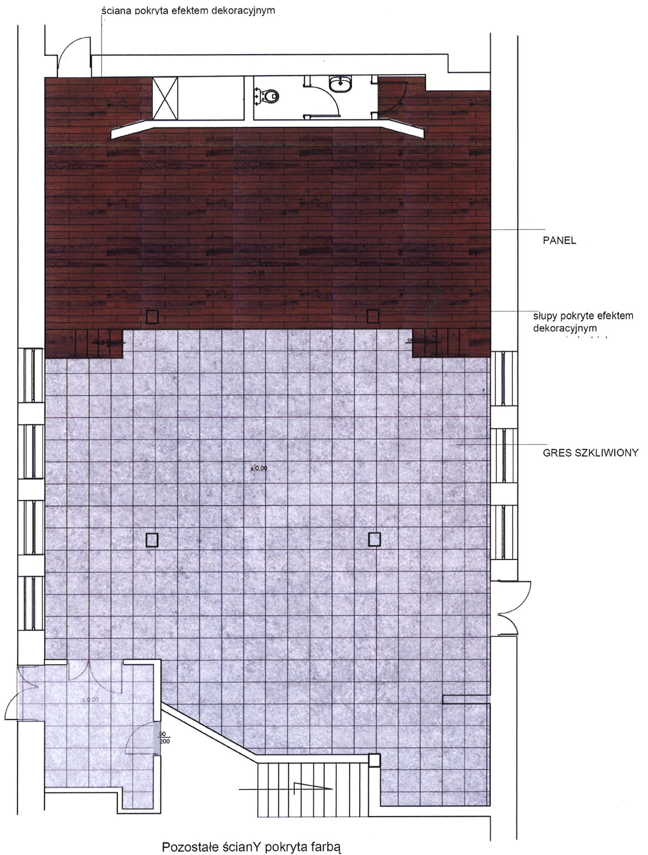
SALA W JAŚWIŁACH RZUT, SKALA 1: 100
